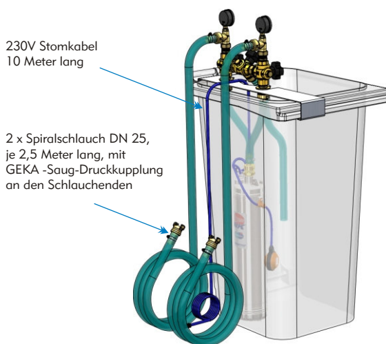
Feine Details III Alles flachdichtend, alles mit dabei...
