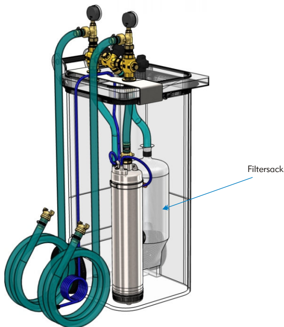
Feine Details I Große Filtersäcke
